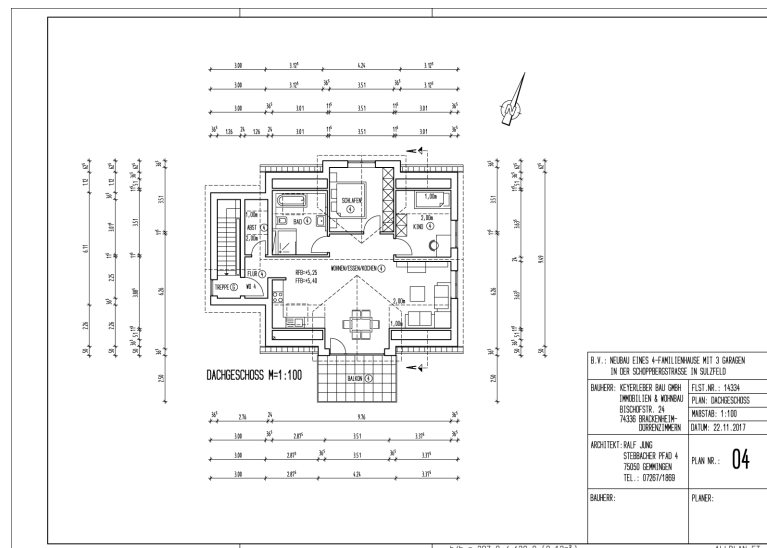
Grundriss Dachgeschoss
