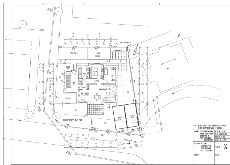
Grundriss Erdgeschoss
