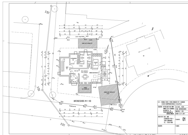
Grundriss Untergeschoss
