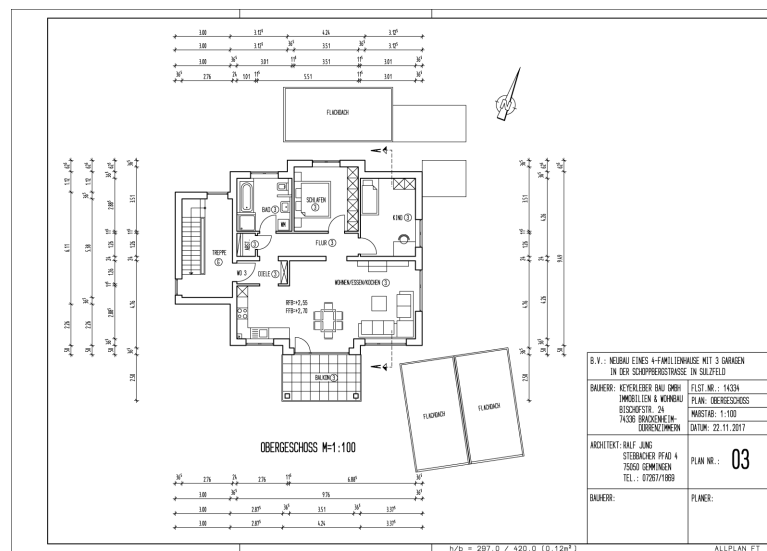
Grundriss Obergeschoss
